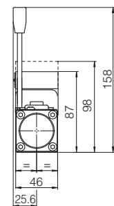
DHZA/*-06*/MV DHZA/UL-*06*/MV (dotted line)
