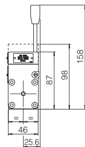
Mass: 3,4 kg
