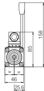
QVHZO-A-06*/MV Mass: 3,2 kg
